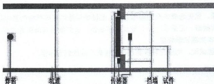
图 A. 3 试验装置示意图(a-a)
