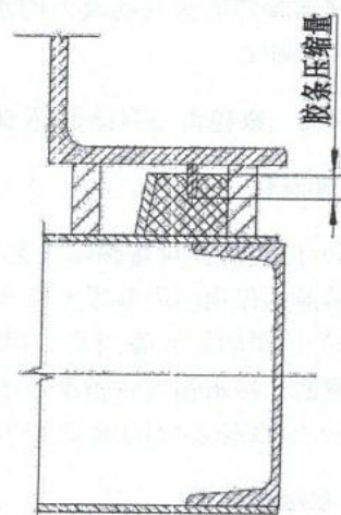
图2 嵌压式
