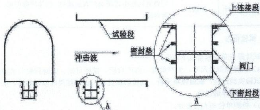
图 B.4 阀门固定方式示意图
