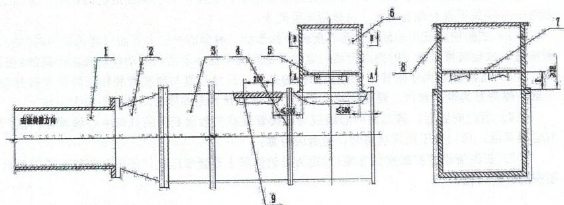
(a) 击波正向进入试验装置
