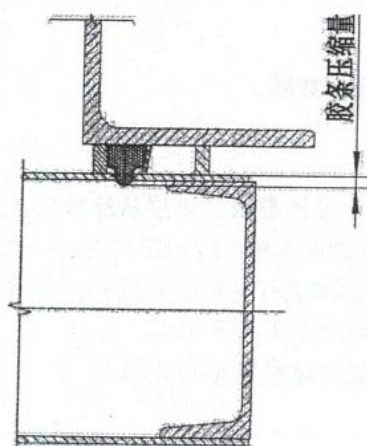
图1 挤压式
