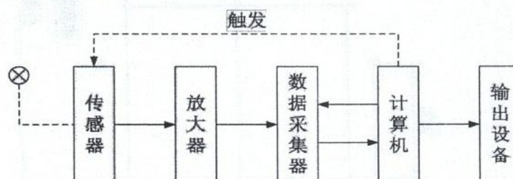
图 A. 1 测试系统工作原理示意图
