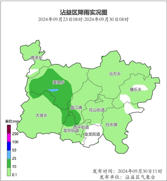
图 1 2024 年 9 月 23 日 08 时至 9 月 30 日 08 累积降雨量（单位：毫米）
